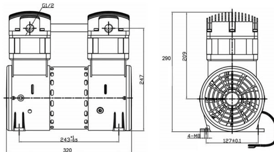
產品尺寸圖
