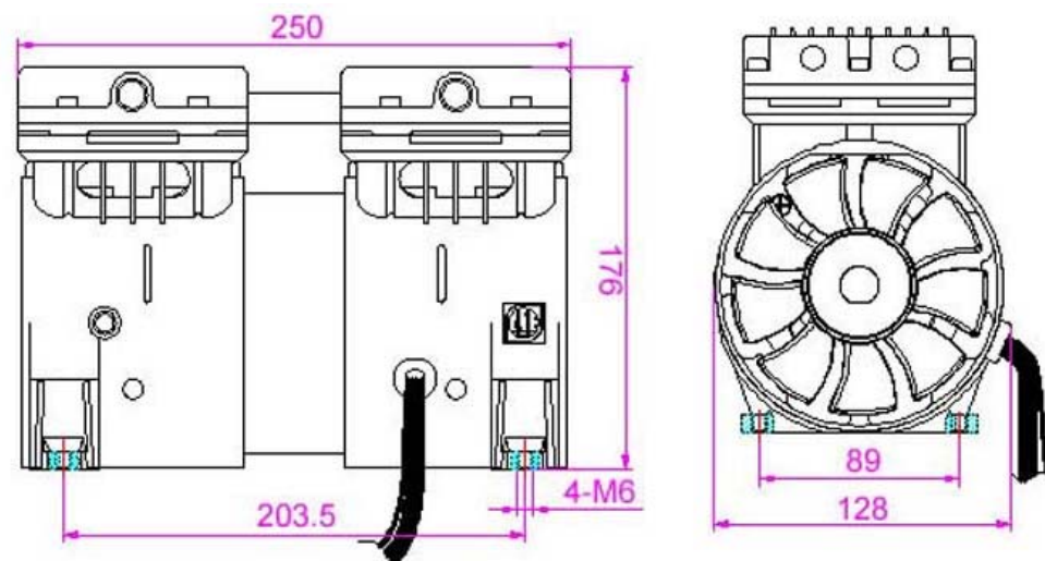
產品尺寸圖
